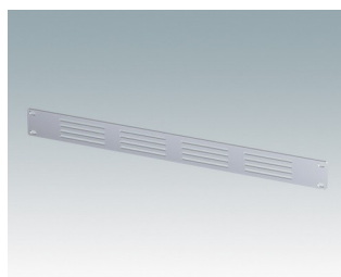
M6019011 Frontplatte 1HEX19" mit Lüftung Aluminium Matt eloxiert 482,6x3x43,6mm
