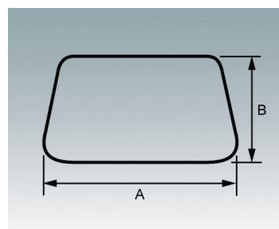
M0000805 Ausschnitt, D-Sub Stanzwerkzeuge
