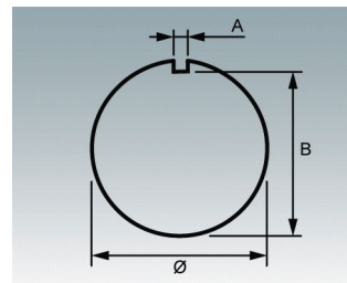
M0000808 Ausschnitt, rund mit Nase Stanzwerkzeuge
